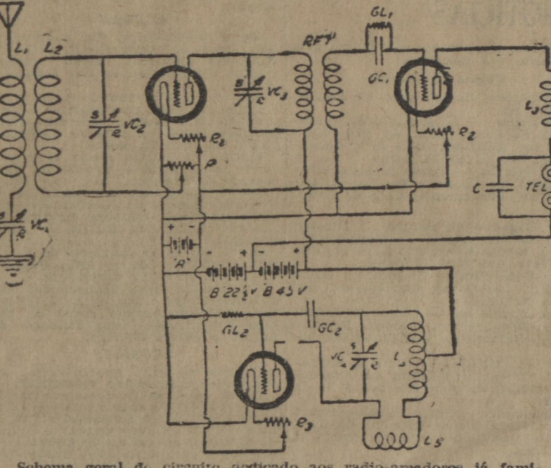
Schema geral do circuito contendo os radio-amadores já familiarizados com a moderna tecnica
